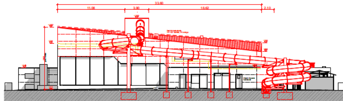
Südost Fassade
