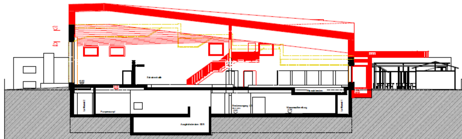
Schnitt Q1 - Q1
