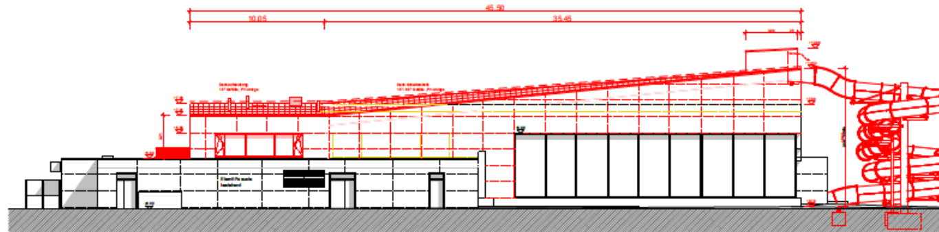
Südwest Fassade
