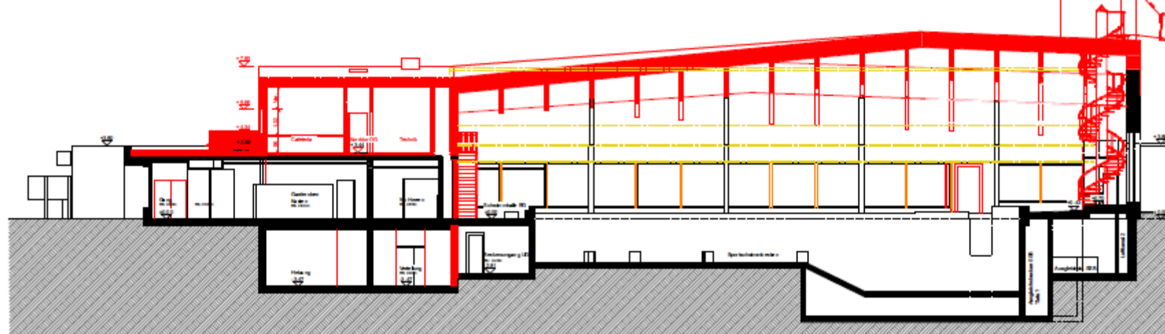
Schnitt L1 - L1
